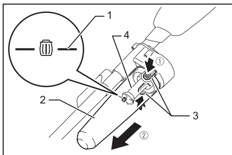
► 1. Linha de enchimento completo 2. Reservatório de pó 3. Botão (dois locais) 4. Filtro de malha
