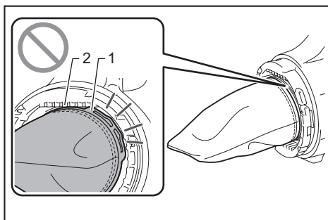
► 1. Borda de fixação 2. Ranhura da caixa do aspirador
