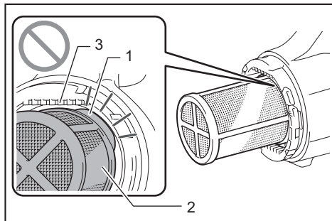
► 1. Borda de fixação 2. Pré-filtro 3. Ranhura da caixa do aspirador
