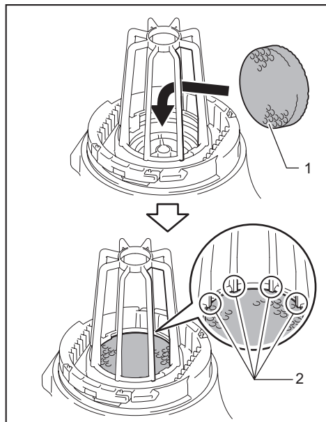
► 1. Filtro de esponja 2. Borda inferior da coluna
