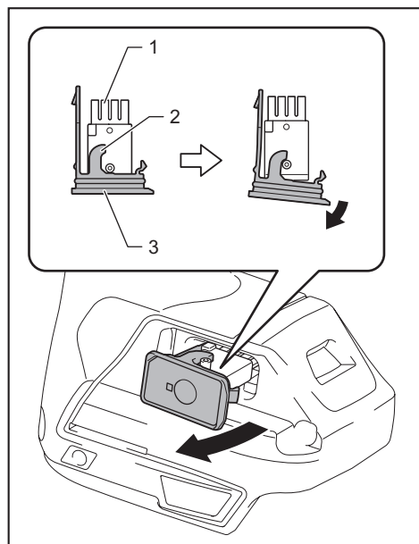
► 1. Unidade de comunicação sem fio 2. Gancho 3. Tampa
