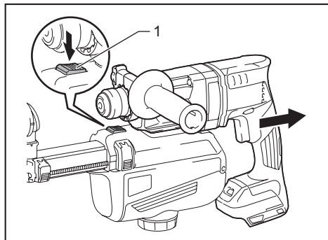
► 1. Botão de liberação da trava
