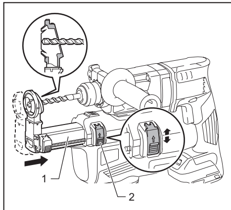
► 1. Guia 2. Botão de ajuste da guia
