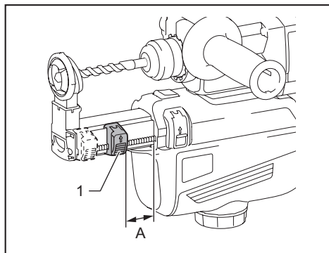
► 1. Botão de ajuste da profundidade
