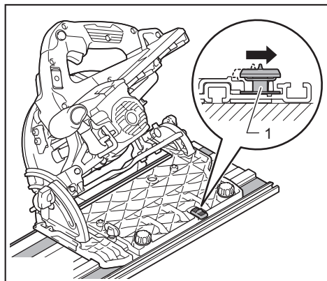
► 1. Alavanca corredeira
