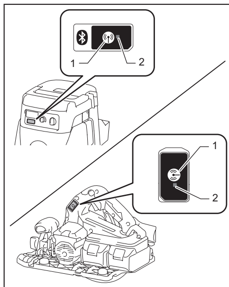
► 1. Botão da ativação sem fio 2. Lâmpada da ativação sem fio
