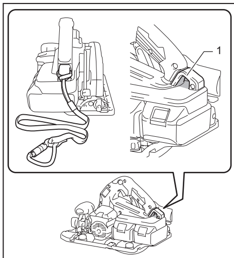
► 1. Furo para o cordão de segurança (correia de retenção)
