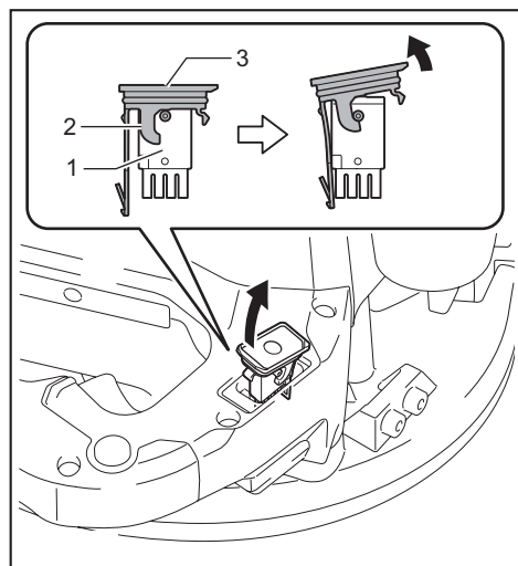
► 1. Unidade de comunicação sem fio 2. Gancho 3. Tampa
