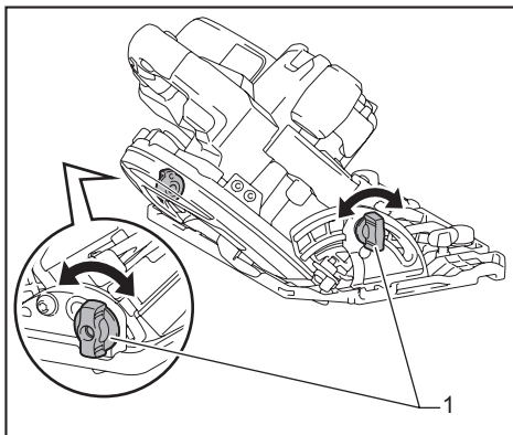
► 1. Parafuso de fixação
