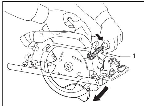
► 1. Alavanca retrátil
