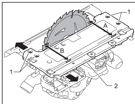
► 1. Parafuso 2. Base
