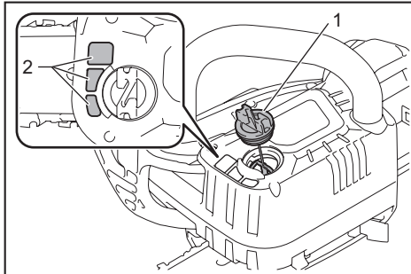
► 1. Tampa do tanque de óleo 2. Visor de inspeção de óleo
