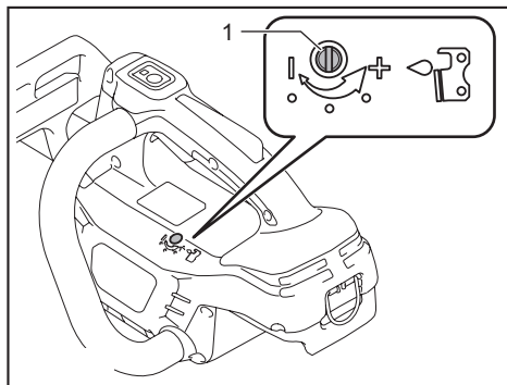
► 1. Parafuso de ajuste
