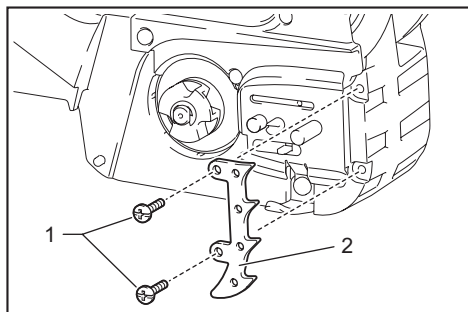
► 1. Parafuso 2. Amortecedor dentado
