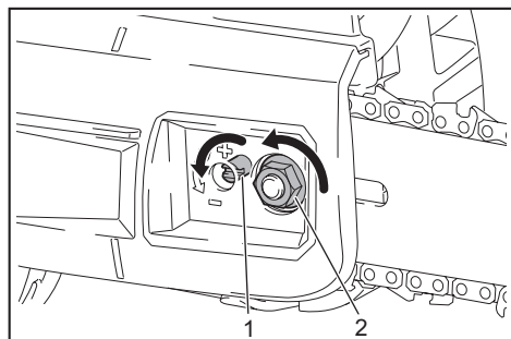
► 1. Parafuso de ajuste da corrente 2. Porca de retenção
