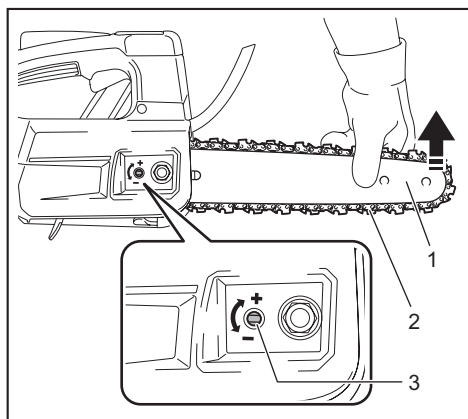
► 1. Sabre 2. Corrente da serra 3. Parafuso de ajuste da corrente
