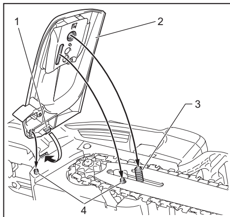
► 1. Ressalto 2. Cobertura da roda dentada 3. Parafuso passante 4. Pino
