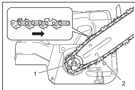
► 1. Roda dentada 2. Furo
