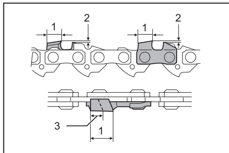
► 1. Comprimento do cortador 2. Distância entre a borda de corte e o limitador de profundidade 3. Comprimento mínimo do cortador (3 mm)
