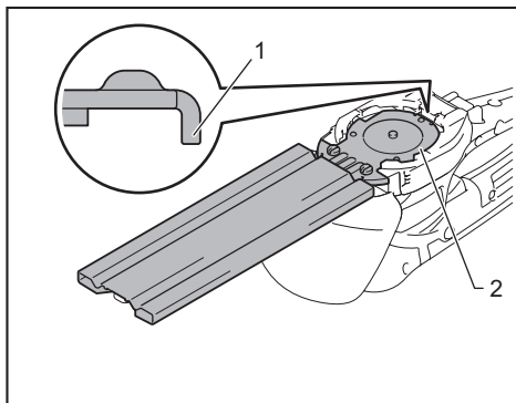
► 1. Garra 2. Placa-guia
