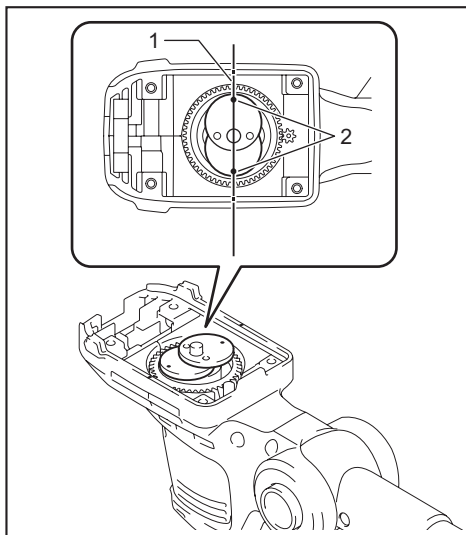
► 1. Linha de alinhamento 2. Furo pequeno
