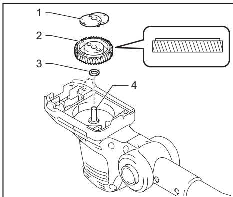
► 1. Manivela 2. Engrenagem 3. Arruela 4. Pino
