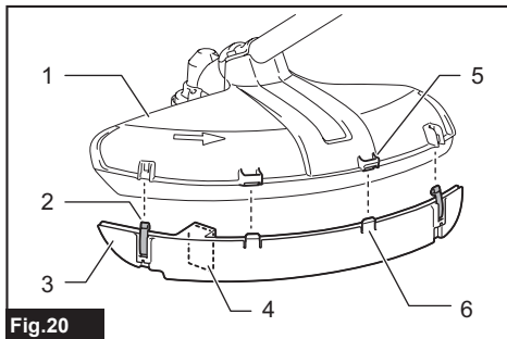
Fig.20 ► 1. Proteção 2. Grampo 3. Extensão da proteção 4. Cortador 5. Encaixe 6. Aba
