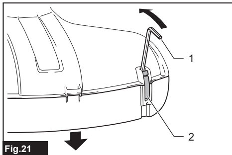
Fig.21 ► 1. Chave sextavada 2. Grampo
