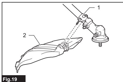
Fig.19 ► 1. Abraçadeira 2. Proteção
