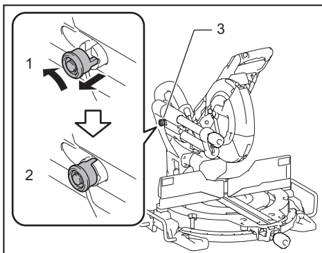
► 1. Posição destravada 2. Posição travada 3. Pino de trava
