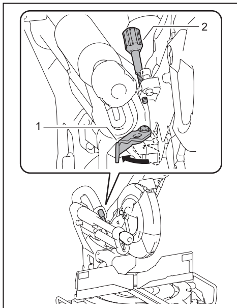
► 1. Placa de retenção 2. Parafuso de ajuste
