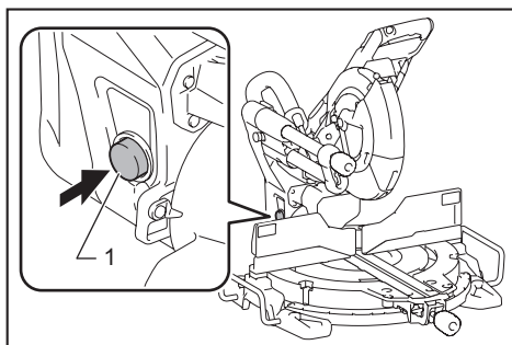
► 1. Botão de liberação
