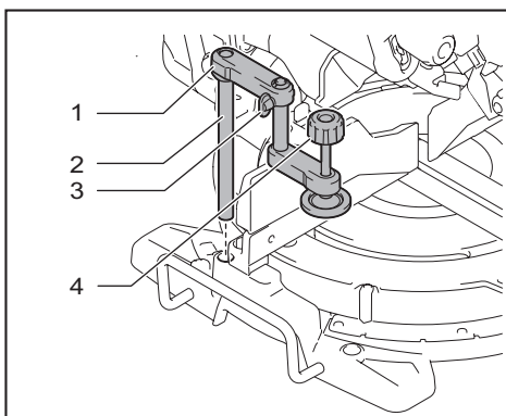
► 1. Braço da morsa 2. Haste da morsa 3. Parafuso de fixação 4. Botão da morsa
