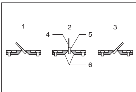
► 1. Corte de bisel à esquerda 2. Corte reto 3. Corte de bisel à direita 4. Disco de corte 5. Dente do disco 6. Placa de corte
