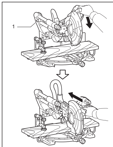
► 1. Pino de trava
