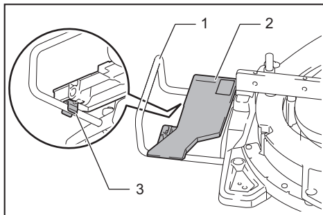
► 1. Suporte 2. Placa superior 3. Grampo
