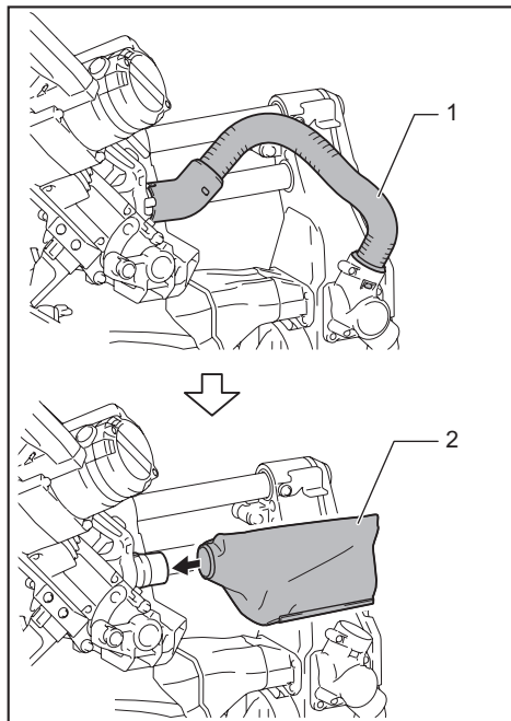
► 1. Mangueira de extração de pó 2. Saco de pó
