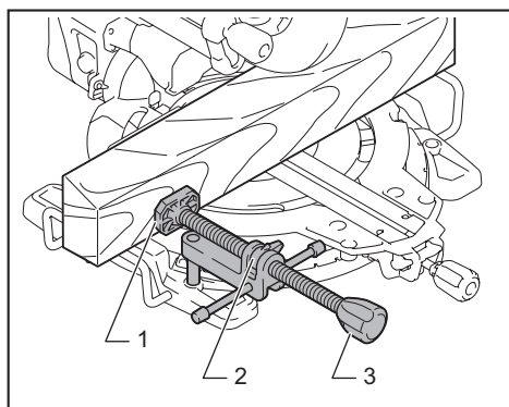
► 1. Placa da morsa 2. Porca da morsa 3. Botão da morsa
