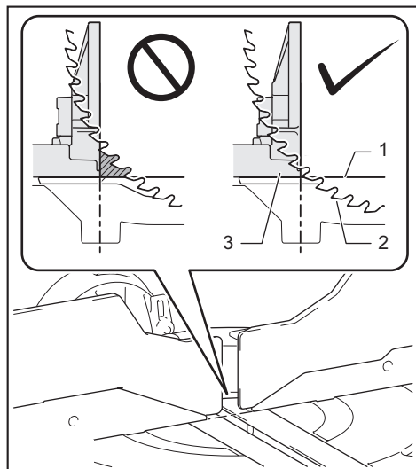
► 1. Superfície superior da base giratória 2. Borda do disco 3. Placa guia
