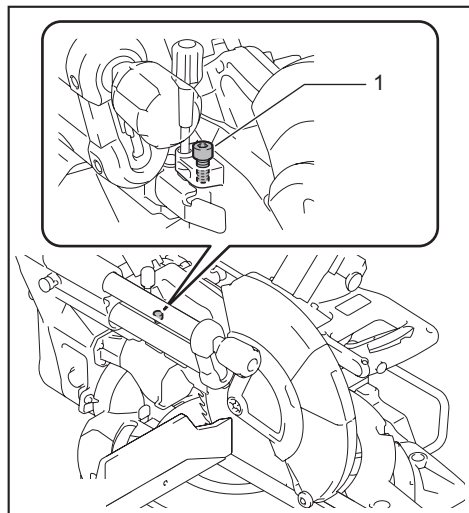
► 1. Parafuso passante de ajuste
