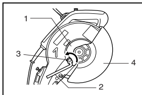
1. Tampa central 2. Chave hexagonal 3. Parafuso hexagonal 4. Protetor de segurança do disco
