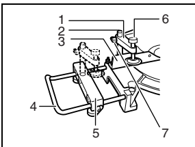
1. Braço da morsa 2. Vareta da morsa 3. Placa guia 4. Suporte 5. Conjunto do suporte 6. Regulador da morsa 7. Parafuso
