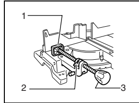
1. Placa da morsa 2. Porca da morsa 3. Regulador da morsa
