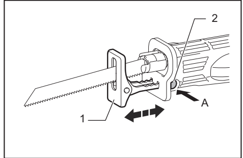
► 1. Sapata 2. Botão da sapata
