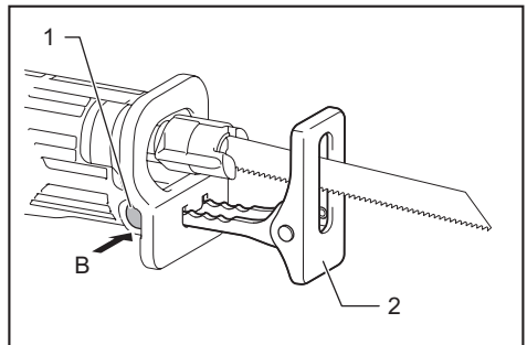
► 1. Botão da sapata 2. Sapata
